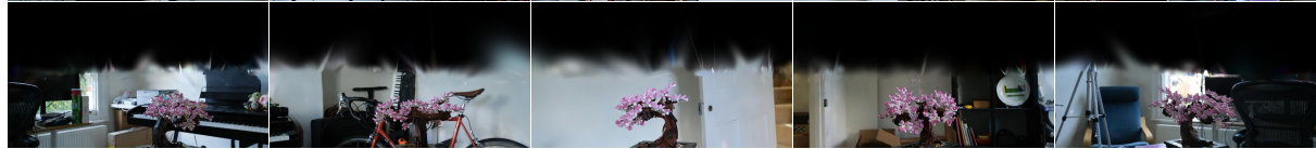
Vanilla 3DGS
